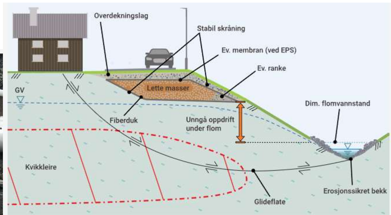
Figur 1: Prinsippskisse for terrengavlasting med bruk av lette masser.
